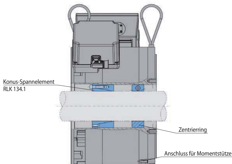
Ausführung Spannsystem RTM 134.1 für eine Spannstelle
