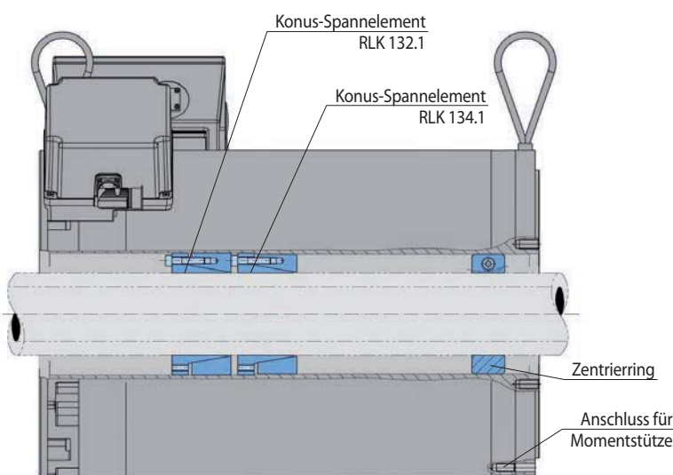
Ausführung Spannsystem RTM 134.2 für zwei Spannstellen
