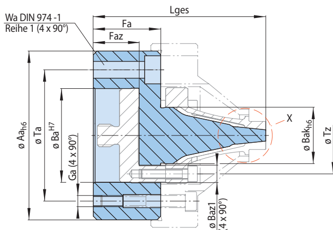
Größe HKDF 4 bis HKDF 7
