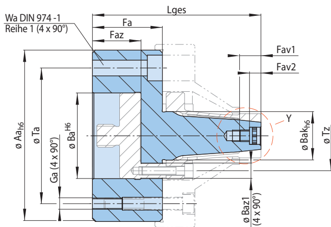
Größe HKDF 12 und HKDF 19 mit Verschlussstopfen
