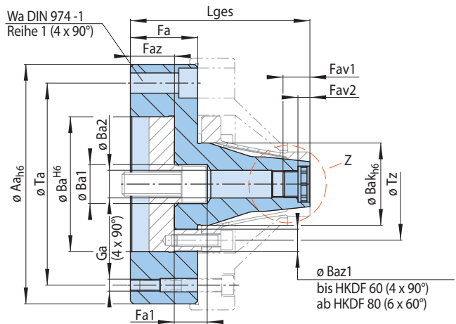
Größe HKDF 30 bis HKDF 125 mit Verschlussstopfen
